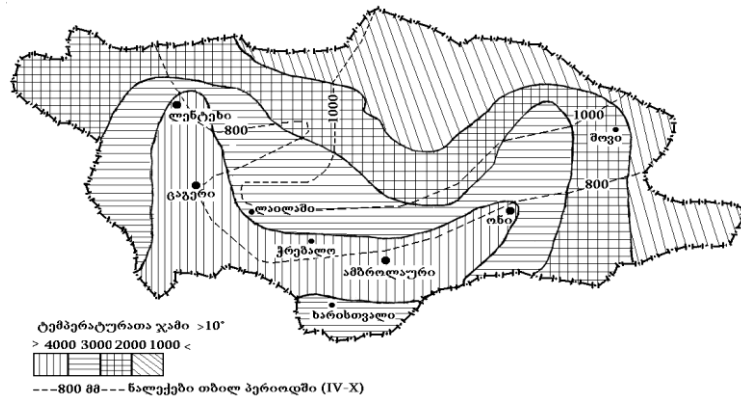
ნახ. 4.2.1 რაჭა-ლენხუმი - ქვემო სვანეთის რეგიონის აგროკლიმატური ზონები:
