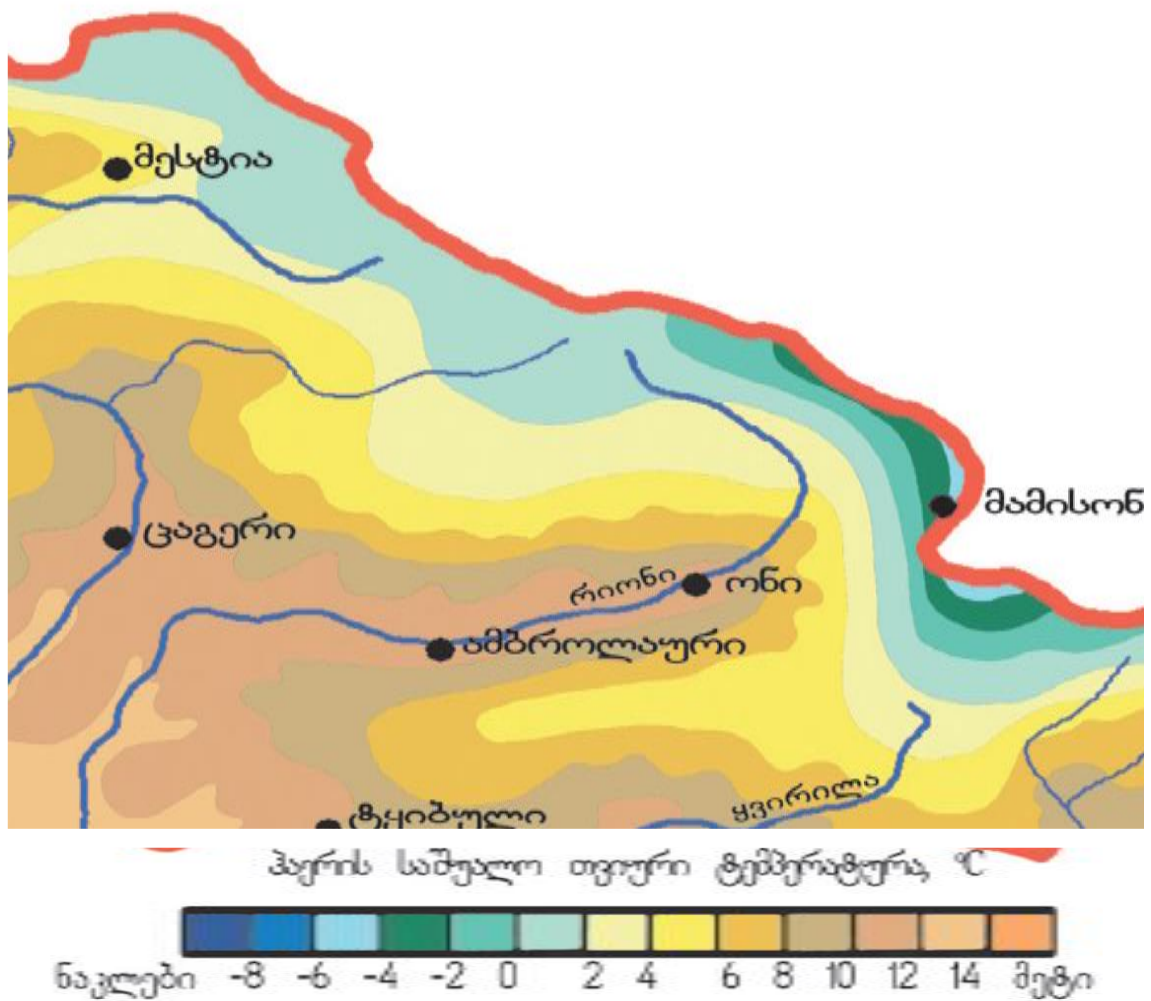
ნახ 2.1.4. პაერის ტემპერატურა (აპრილი)
