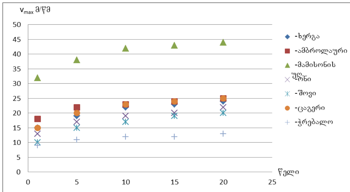
ნახ. 5.1.1. ქარის მაქსიმალური სიჩქარე შესაძლო ერთხელ 1,5,10,15 და 20 წლის გამნავლობაში. ◆-ხერგა, ■-ამბროლაური, ▲-მამოსონის უღელტეხილი, ×-ონი, * -შოვი, ●-ცაგერი, + -ჭრებალო.
