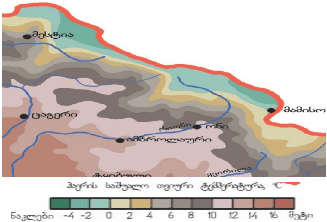
ნახ. 2.1.6. ჰაერის ტემპერატურა (ოქტომბერი)
