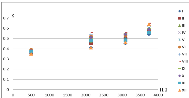
ნახ. 1.2.1 დრუბლიანობის კოეფიციენტის დამოკიდებულება ადგილის აბსოლუტურ სიმაღლეზე K=f(H)
