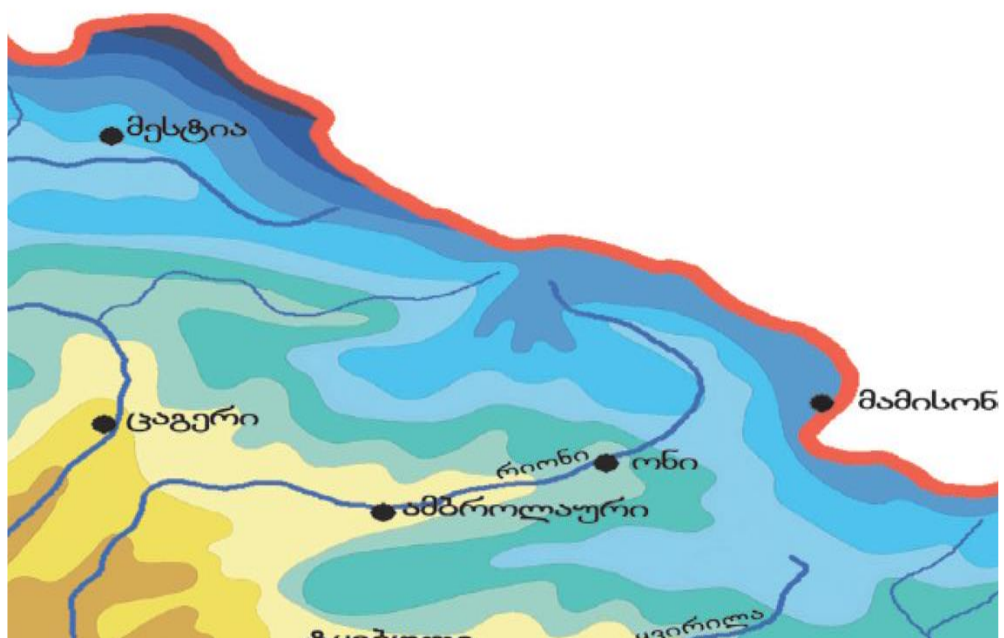
ჰაერის საშუალო თვიური ტემპერატურა, °C ნაკლები -14 -12 -10 -8 -6 -4 -2 0 2 4 5 6 მეტი
