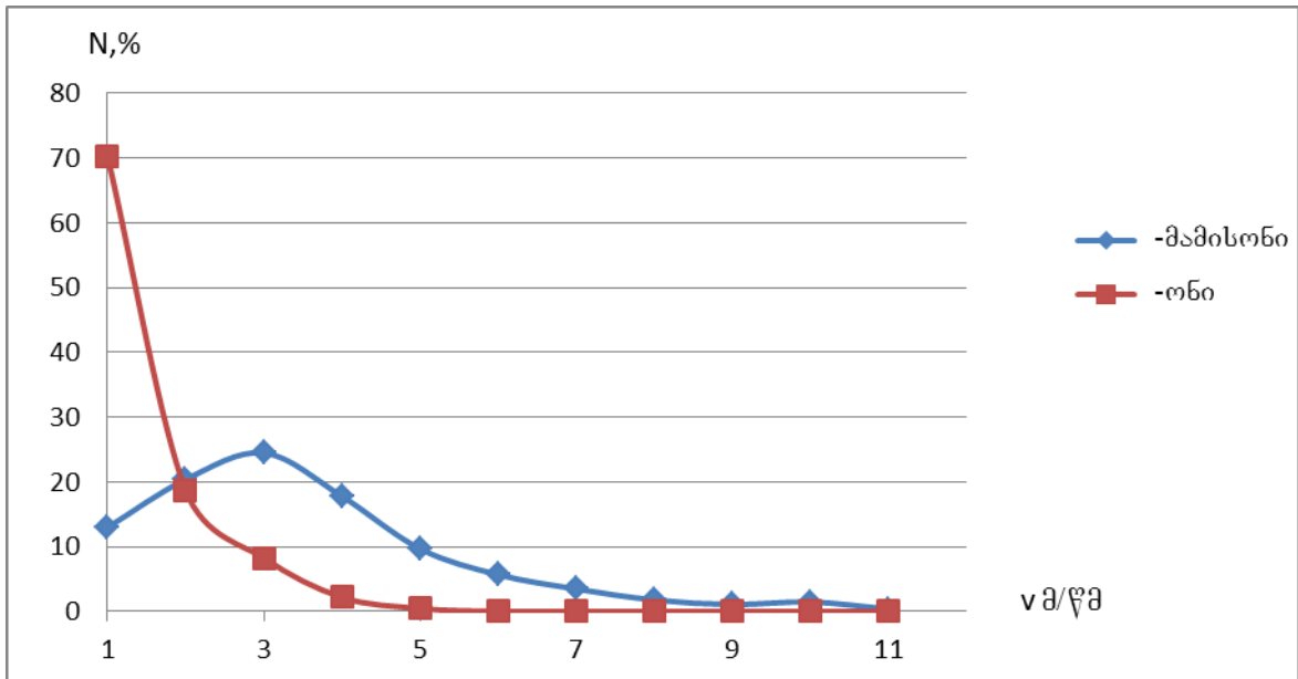
ნახ. 2.5.2. ქარის სიჩქარის განმეორადობა გრადაციების მიხედვით, %
