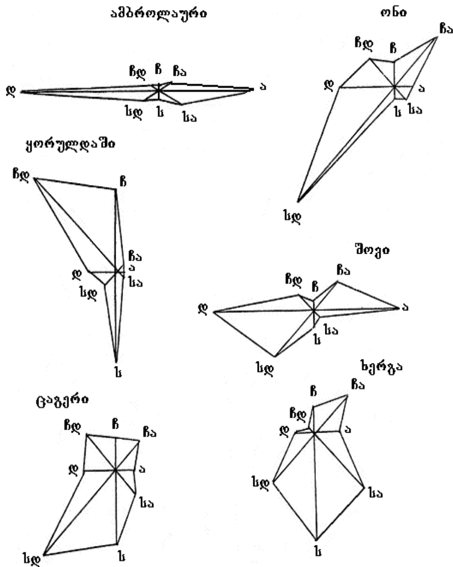
ნახ. 4.3.1 გაბატონებული ქარების მიმართულებების განმეორადობა (%) თბილ პერიოდში
