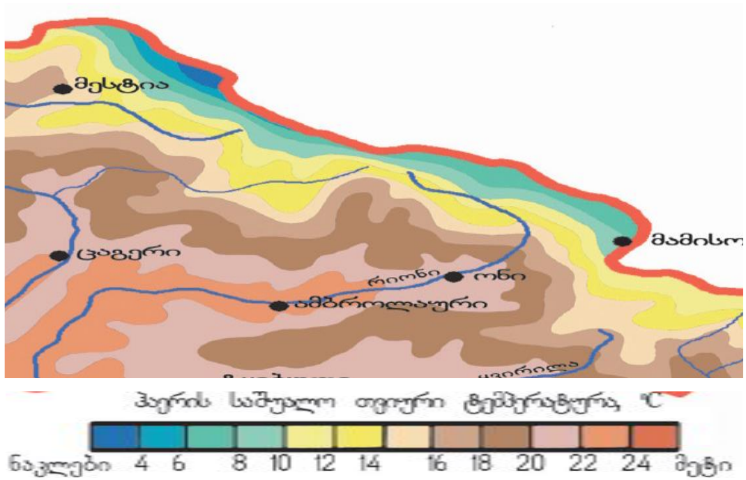
ნახ. 2.1.5. ჰაერის ტემპერატურა (ივლისი)
