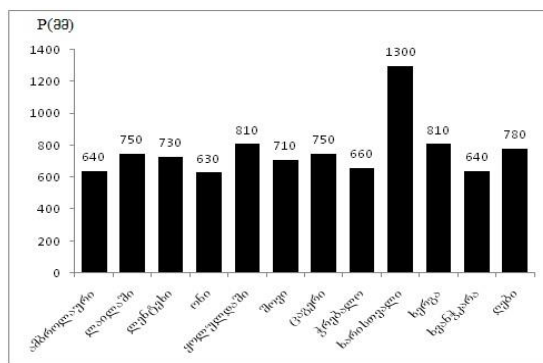
ნახ. 4.1.3. რაჭა-ლეჩხუმი - ქვემო სვანეთის რეგიონის ატმოსფერული ნალექების ჯამები (მმ) თბილ პერიოდში
