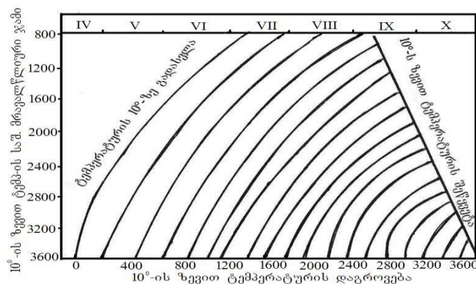
ნახ. 4.1.2 ჰაერის ტემპერატურათა (10°C-ის ზევით) ჯამის დაგროვება დამოკიდებული ტემპერატურის საშუალო მრავალწლიურ ჯამზე
