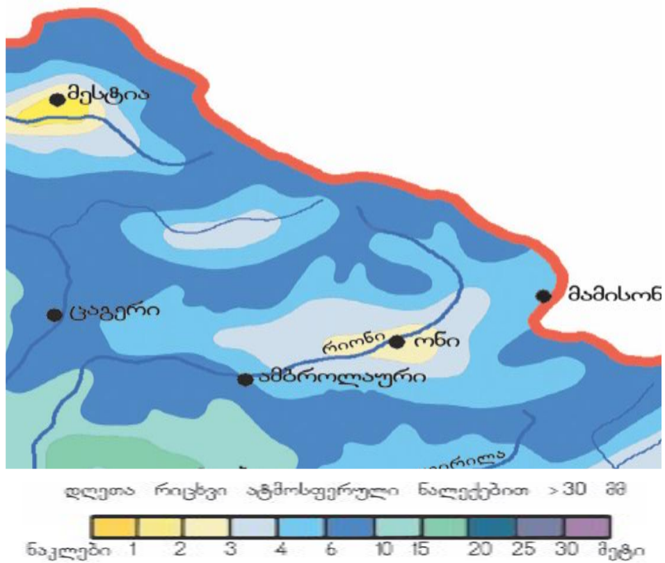
ნახ. 5.5.1. დღეთა რიცხვი უხვი ნალექებით წელიწადში
