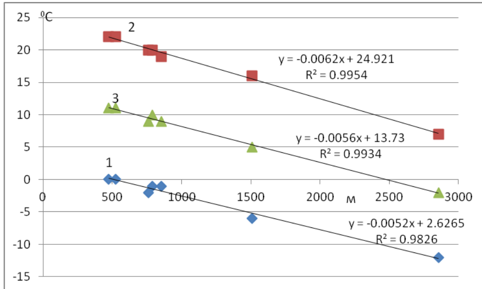
ნახ. 2.1.1. ჰაერის ტემპერატურის ცვლილება სიმაღლის მიხედვით რაჭა-ლეჩხუმი, ქვემო სვანეთის რეგიონში და შესაბამისი აღმწერი ფუნქციები: 1-იანგარი; 2-ივლისი; 3-წელი ( R^2 -დეტერმინაციის კოეფიციენტი)
