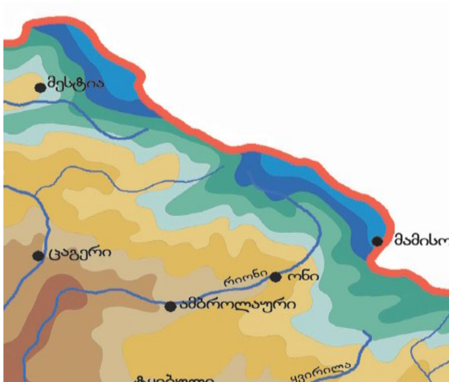
ჰაერის საშუალო წლიური ტემპერატურა, °C ნაკლები -6 -4 -2 0 2 4 6 8 10 12 14 მეტი
