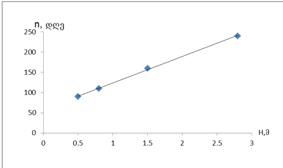
ნახ.2.4.1. თოვლის საფარის ხანგრძლივობის დამოკიდებულება ადგილის აბსოლუტურ სიმაღლეზე, n=f(H)
