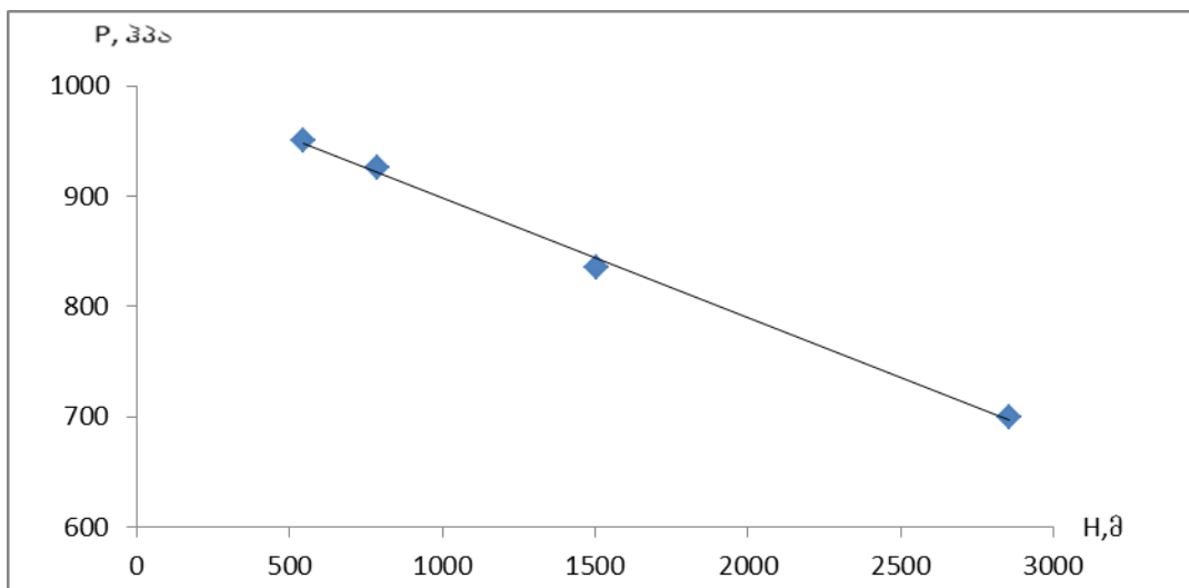
ნახ. 1.3.1. დამოკიდებულება P=f(H)
