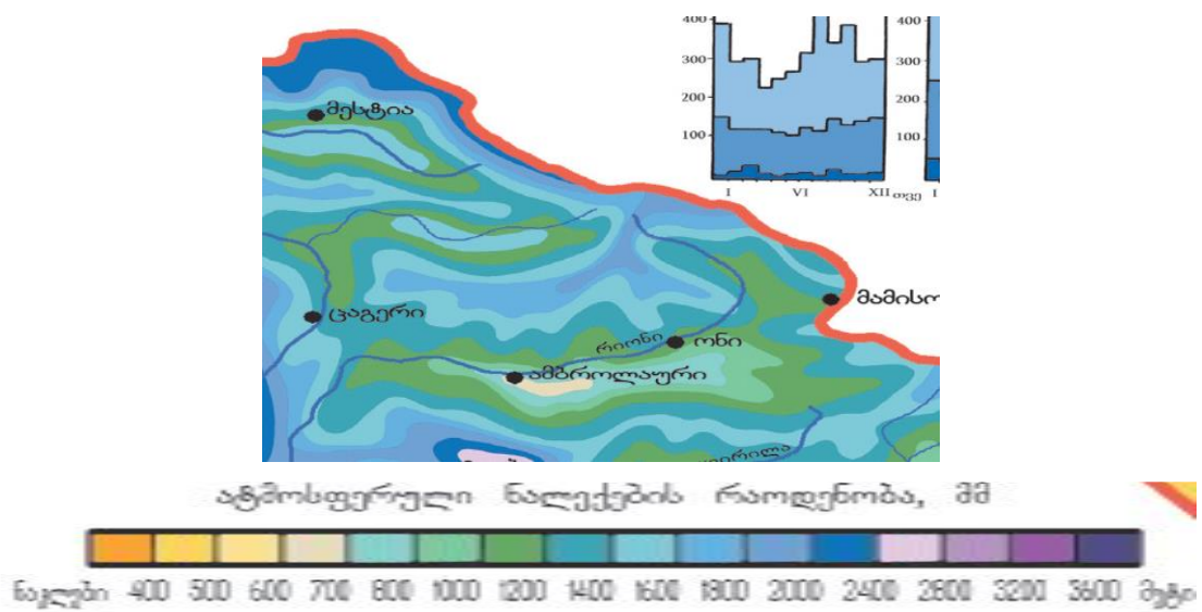
ნახ. 2.3.3. ატმოსფერული ნალექების წლიური ჯამები (მმ)
