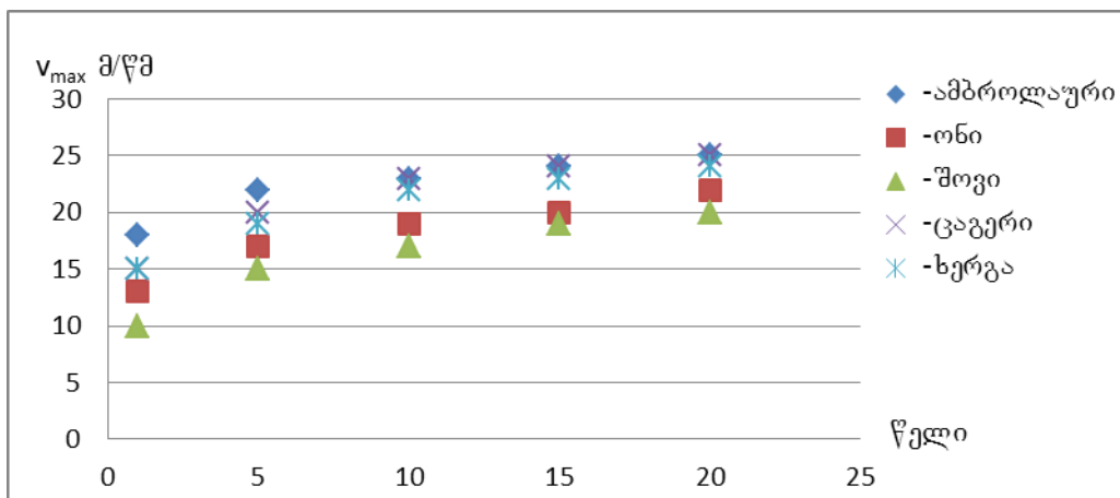
ნახ. 2.5.1. ქარის მაქსიმალური სიჩქარის ( V_{max} ) დამოკიდებულება წლების რაოდენობაზე
