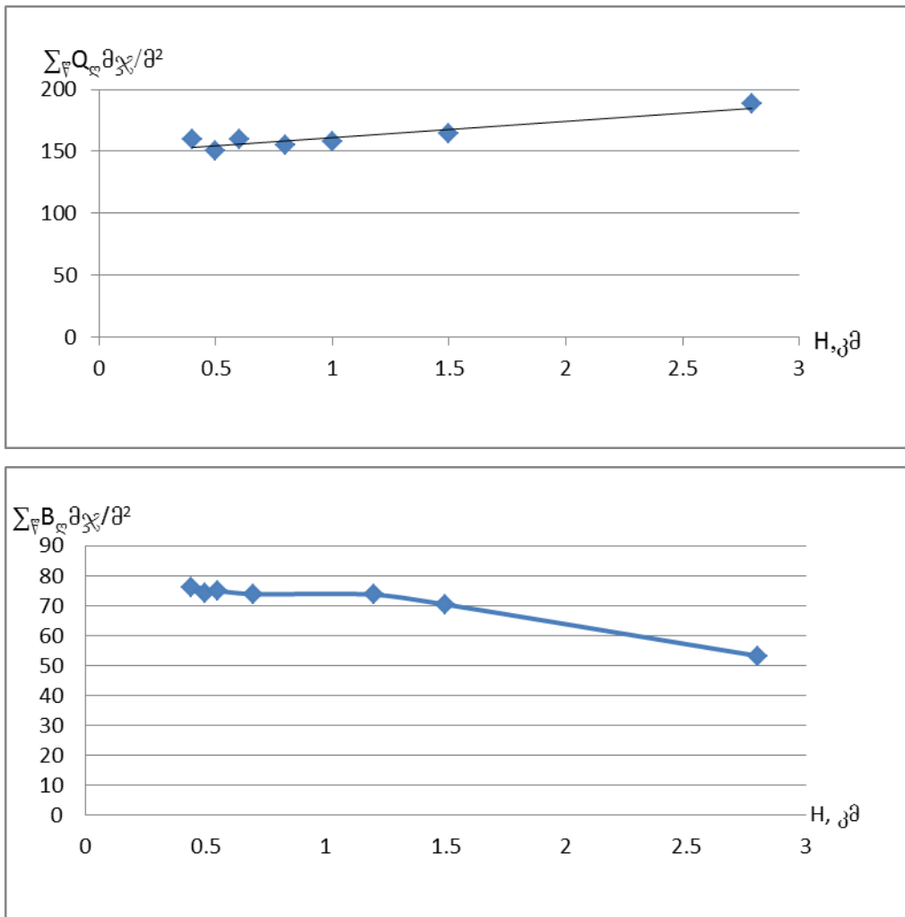
ნახ.1.2.2. დამოკიდებულებები \Sigma_{\text{წ}}Q_{\text{ღ}} = f(H) და \Sigma_{\text{წ}}B_{\text{ღ}} = f(H)
