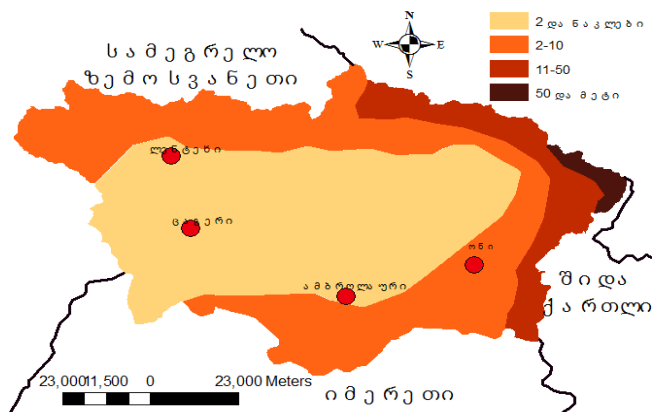
ნახ.5.2.1 ქარბუქიან დღეთა საშუალო წლიური რიცხვი
