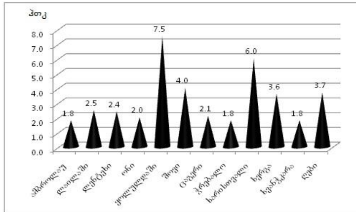
ნახ. 4.1.4 რაჭა-ლეჩხუმი - ქვემო სვანეთის რეგიონის ჰიდროთერმული კოეფიციენტის მაჩვენებლები თბილ პერიოდში
