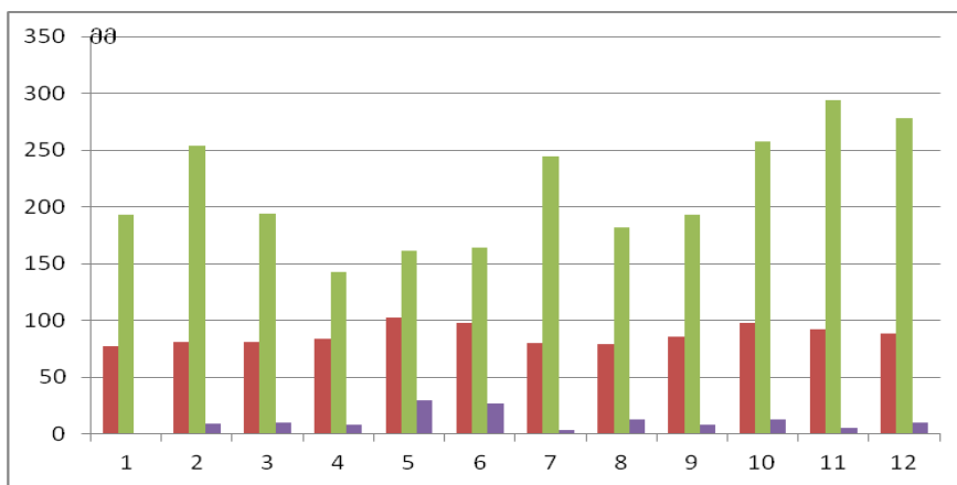
ნახ. 2.3.1. ატმოსფერული ნალექების წლიური სველა ონში: უდიდესი, საშუალო და უმცირესი მნიშვნელობები
