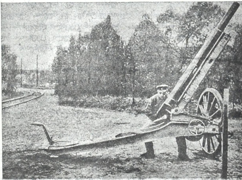
გერმანული ზარბაზანი ჰაეროპლანების და ჰაერის გემთა საწი-ნალმდეგოდ.
