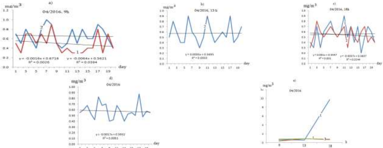
ნახ. 6. მტერის კონცენტრაციის მნიშვნელობები № 6 და № 2 სადამკვირვებლო პუნქტებში 9 (a), 13 (b) და 18 (c) სთ-ზე; საშუალო დღიური კონცენტრაციები (d); მტერის კონცენტრაცია 9 (a), 13 (b) და 18 (c) სთ-ზე თვის 5(1), 15(2) და 25(3) რიცხვებში (e); ტრენდის განტოლებები, გრაფიკები და დისპერსიის მნიშვნელობები 2016 წლის აპრილში
