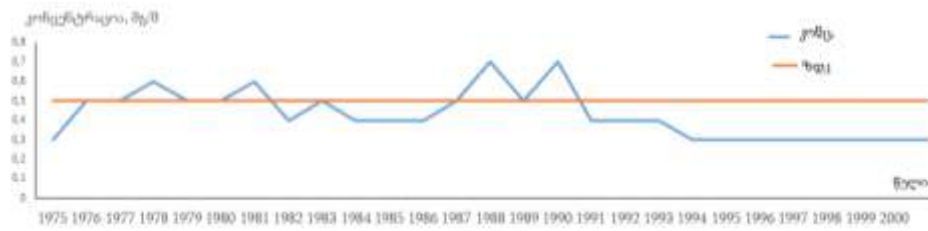
ნახ. 1. ქ.თბილისის ატმოსფეროში მტვრის საშუალო წლიური კონცენტრაციის მნიშვნელობები (მგ/მ³)
