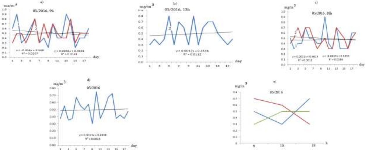
ნახ. 7. მტერის კონცენტრაციის მნიშვნელობები № 6 და № 2 სადამკვირვებლო პუნქტებში 9 (a), 13 (b) და 18 (c) სთ-ზე; საშუალო დღიური კონცენტრაციები (d); მტერის კონცენტრაცია 9 (a), 13 (b) და 18 (c) სთ-ზე თვის 5(1), 15(2) და 25(3) რიცხვებში (e); ტრენდის განტოლებები, გრაფიკები და დისპერსიის მნიშვნელობები 2016 წლის მაისში
