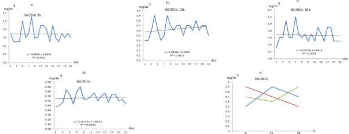
ნახ. 8. მტერის კონცენტრაციის მნიშვნელობები № 6 სადამკვირვებლო პუნქტში 9 (a), 13 (b) და 18 (c) სთ-ზე; საშუალო დღიური კონცენტრაციები (d); მტერის კონცენტრაცია 9 (a), 13 (b) და 18 (c) სთ-ზე თვის 5(1), 15(2) და 25(3) რიცხვებში (e); ტრენდის განტოლებები, გრაფიკები და დისპერსიის მნიშვნელობები 2016 წლის ივნისში
