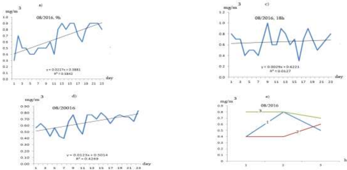
ნახ. 10. მტვრის კონცენტრაციის მნიშვნელობები № 6 სადამკვირვებლო პუნქტში 9 (a) და 18 (c) სთ-ზე; საშუალო დღიური კონცენტრაციები (d); მტვრის კონცენტრაცია 9 (a), 13 (b) და 18 (c) სთ-ზე თვის 5(1), 15(2) და 25(3) რიცხვებში (e); ტრენდის განტოლებები, გრაფიკები და დისპერსიის მნიშვნელობები 2016 წლის აგვისტოში
