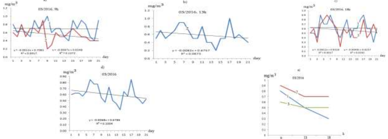
ნახ. 5. მტვრის კონცენტრაციის მნიშვნელობები № 6 და № 2 სადამკვირვებლო პუნქტებში 9 (a), 13 (b) და 18 (c) სთ-ზე; საშუალო დღიური კონცენტრაციები (d); მტვრის კონცენტრაცია 9 (a), 13 (b) და 18 (c) სთ-ზე თვის 5(1), 15(2) და 25(3) რიცხვებში (e); ტრენდის განტოლებები, გრაფიკები და დისპერსიის მნიშვნელობები 2016 წლის მარტში
