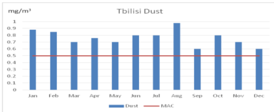
ნახ. 2. ქ.თბილისში მტვრის საშუალო თვიური კონცენტრაციები 2015წ. (www.nea.gov.ge, გარემოს დაბინძურება, ჰაერის წელიწადული-2015)
