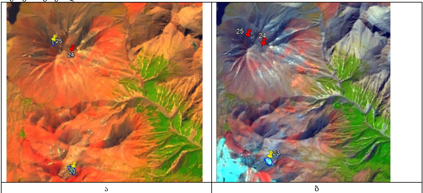
სურ. 3. მდ. მტკვრის მარცხენა შენაკადის, თეთრი არაგვის აუზში მდებარე მცირეები №23-26 მცირეების ვიზუალიზაცია და კონტურები განსაზღვრული Landsat-ის თანამგზავრული სურათის მიხედვით: ა – თდზ 1; ბ – თდზ 2
