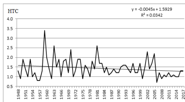
ნახ.1 აქტიურ ტემპერატურათა ( >10^{\circ}\text{C} ) და ატმოსფერული ნალექების (მმ) ჯამების და ჰოკ-ს მსვლელობის დინამიკა (მთიანი ზონა, დმანისი)
