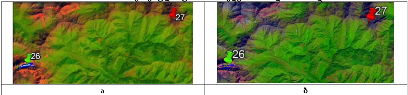
სურ. 4. მდ. მტკვრის მარცხენა შენაკადის, ხევსურეთის არაგვის მარჯვენა შენაკადის აბუდელაურის ხეობაში მდებარე №26 აბუდელაურის და №27 მცირეების ვიზუალიზაცია და კონტურები განსაზღვრული Landsat-ის თანამგზავრული სურათის მიხედვით: ა – თდზ 1; ბ – თდზ 2
