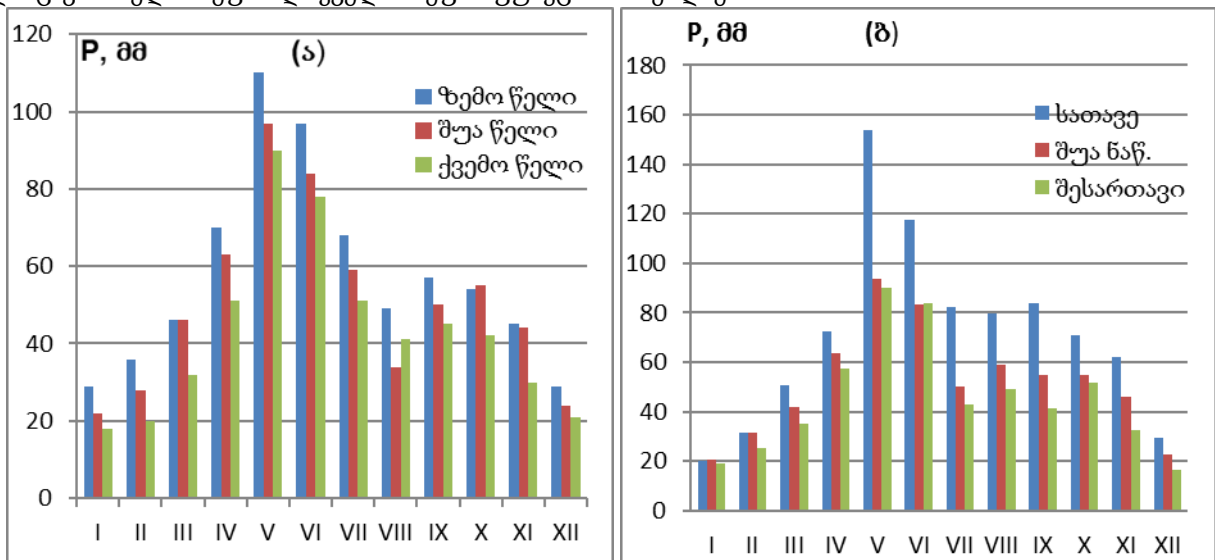
ნახ. 3. ნალექთა ჯამების საშუალო მნიშვნელობები (მმ) იორის აუზის სხვადასხვა მონაკვეთისთვის (ა) კლიმატური ცნობარისა და (ბ) სატელიტური მონაცემების (1986-2018 წწ) მიხედვით [9].
