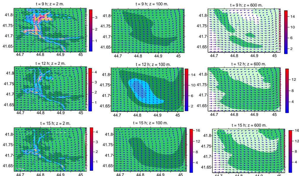
ნახ. 2. ფდ სუსტი ქარის დროს ქარის სიჩქარისა (მ/წმ) და მტვრის კონცენტრაციის (ზდკ) განაწილება, როცა t = 9, 12 და 15 სთ მიწის ზედაპირიდან 2, 100 და 600 მ სიმაღლეებზე
