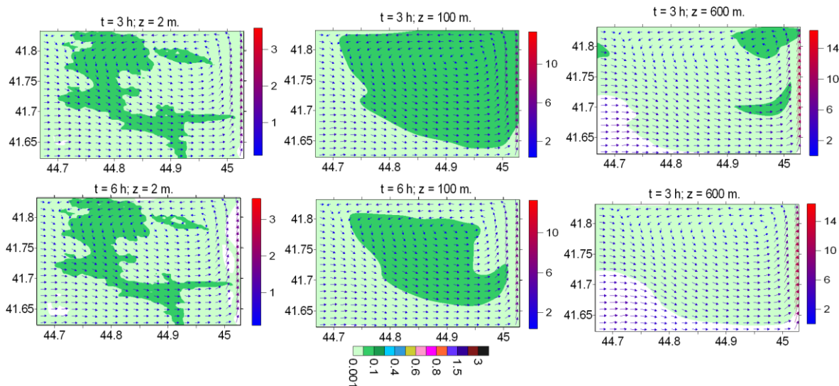
ნახ. 1. ფდ სუსტი ქარის დროს სიჩქარისა ( \text{მ/წმ} ) და მტვრის კონცენტრაციის ( \text{ზდკ} ) განაწილება, როცა t = 3 და 6 სთ მიწის ზედაპირიდან 2, 100 და 600 მ სიმაღლეებზე
