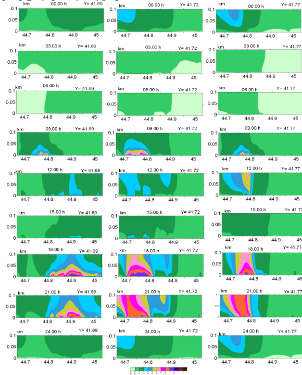
ნახ. 8. ფდ სუსტი ქარის დროს ერთი დღე-ღამის განმავლობაში მტვრის კონცენტრაციების (ზღვ) განაწილება ატმოსფეროს მიწისპირა ფენაში პარალელის გასწვრივ მდებარე სამ ვერტიკალურ სიბრტყეში ( Y = 41.69^{\circ} , Y=41.72^{\circ} და Y=41.77^{\circ} )
