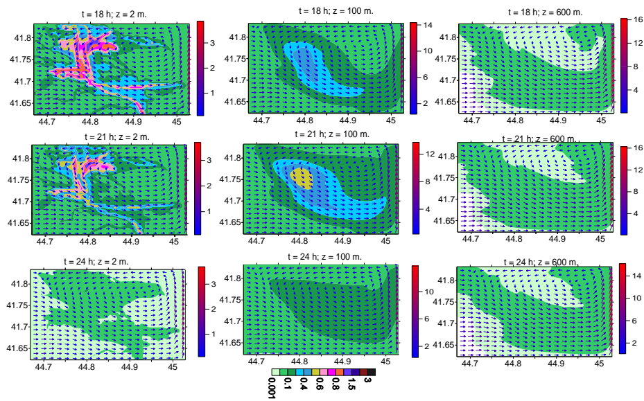
ნახ. 3. ფდ სუსტი ქარის დროს ქარის სიჩქარისა (მ/წმ) და მტვრის კონცენტრაციის (ზდკ) განაწილება, როცა t = 18, 21 და 24 სთ მიწის ზედაპირიდან 2, 100 და 600 მ სიმაღლეებზე
