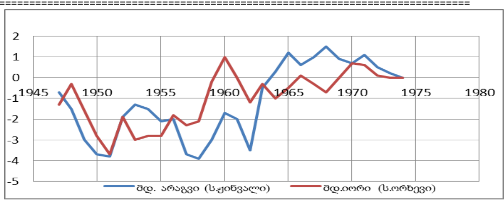
ნახ. 1. მდ არაგვისა და იორის წლიური ჩამონადენის ინტეგრალური მრუდები
